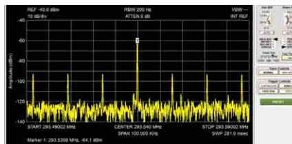
Спектрограмма ПЭМИ видеокамеры
